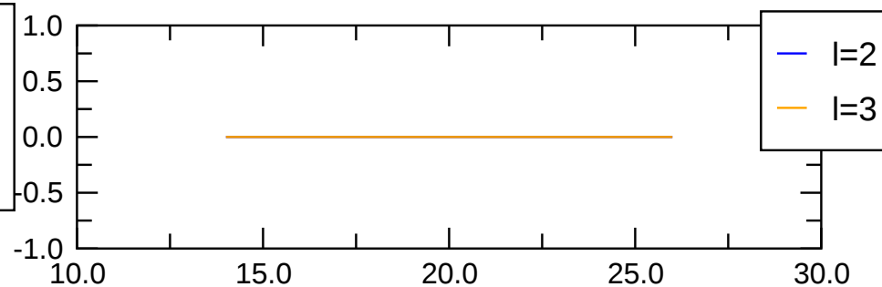
pol(m=0) magn.
