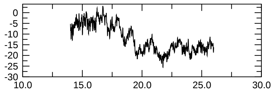
m=2 kin.
