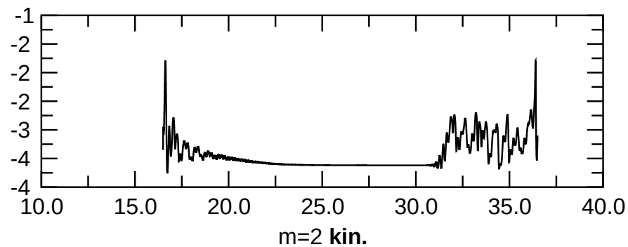
tor(l=1,m=0) kin.
