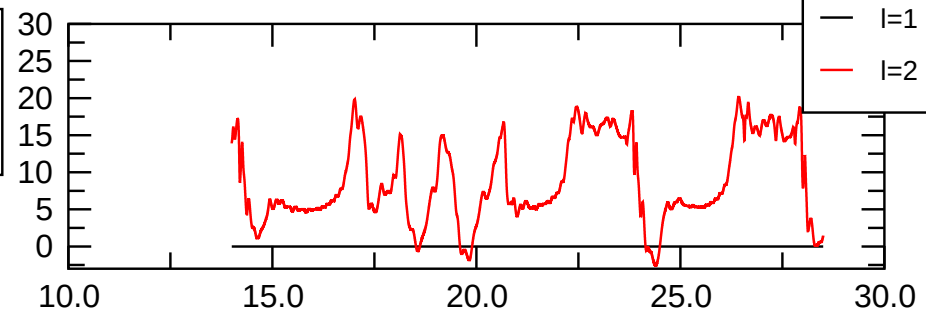
pol(m=2) magn.
