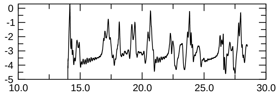
m=2 kin.
