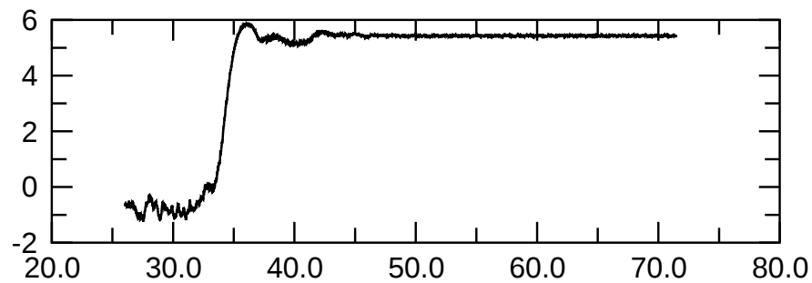
m=2 kin.
