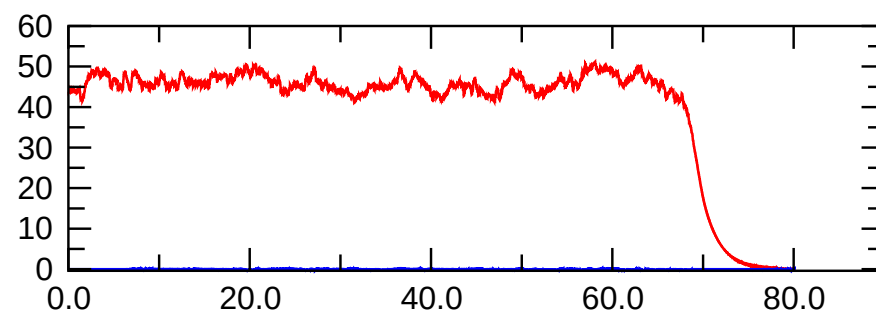
pol(m=0) magn.
