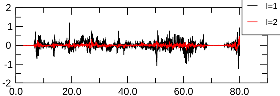
pol(m=2) magn.
