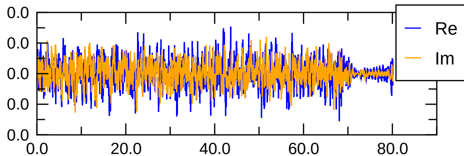
pol(m=1) magn.
