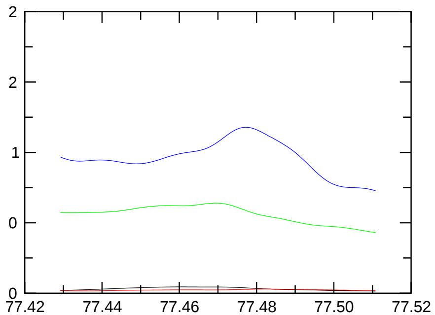
E_{\text{magn,quadr.}}
