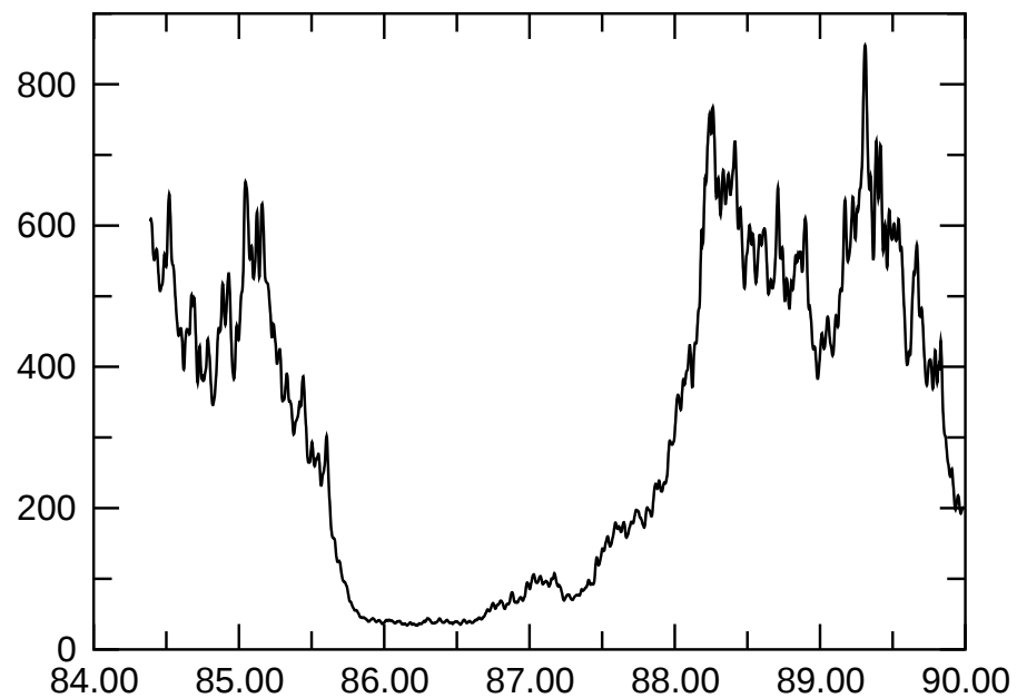
E_{\text{magn,quadr.}}
