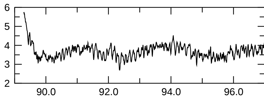
tor( l=1, m=0 ) kin.
