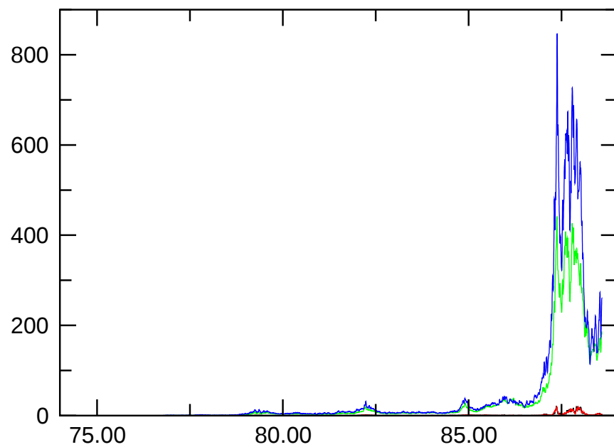
E_{\text{magn,quadr.}}
