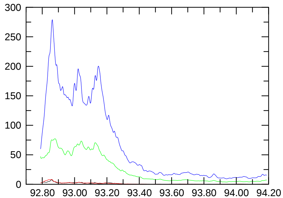
E_{\text{magn,quadr.}}
