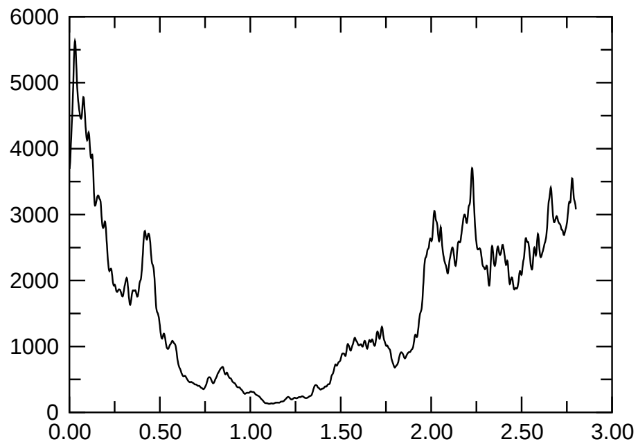
e065p1t2r150000m1p4.5mvbcsolrot1 E_{\text{magn}}
