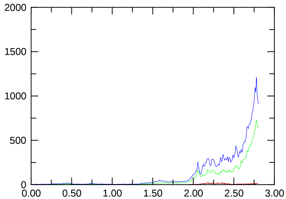
E_{\text{magn,quadr.}}
