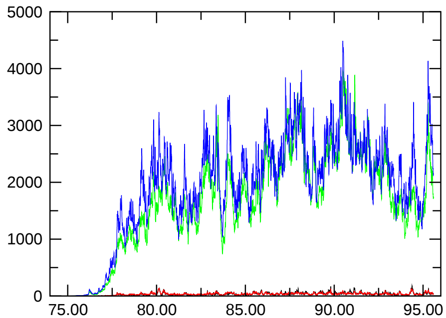
E_{\text{magn,quadr.}}
