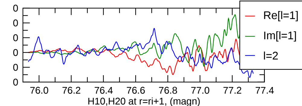
pol( m=1 ) magn.
