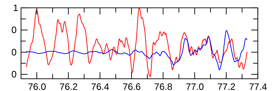
pol( m=0 ) magn.
