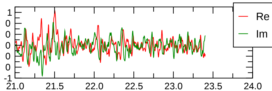
pol( l=1, m=1 ) kin.
