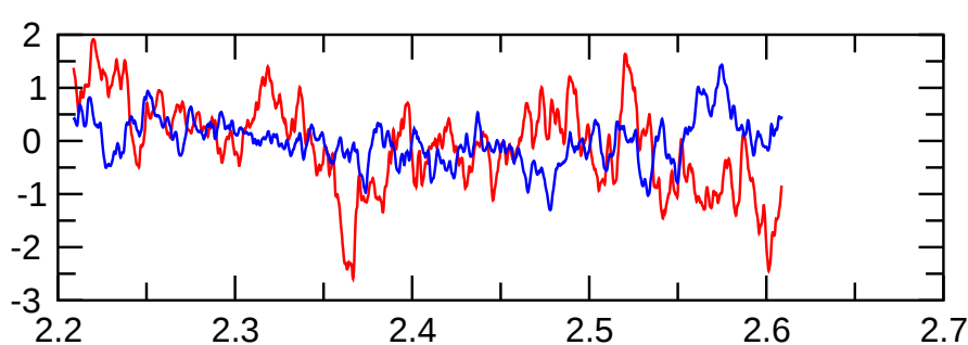
pol(m=0) magn.
