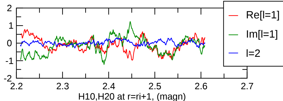
pol(m=1) magn.
