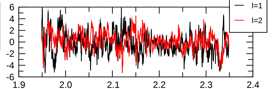
pol(m=2) magn.
