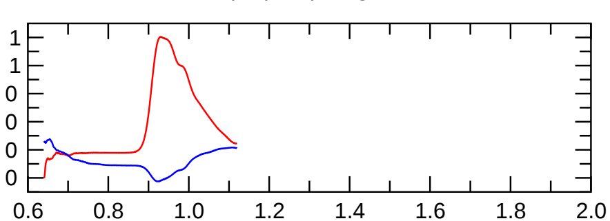
pol(m=0) magn.
