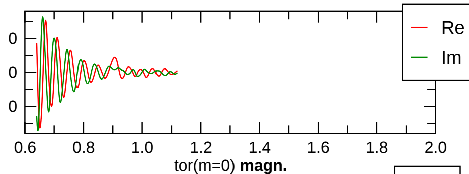
pol(l=1,m=1) kin.
