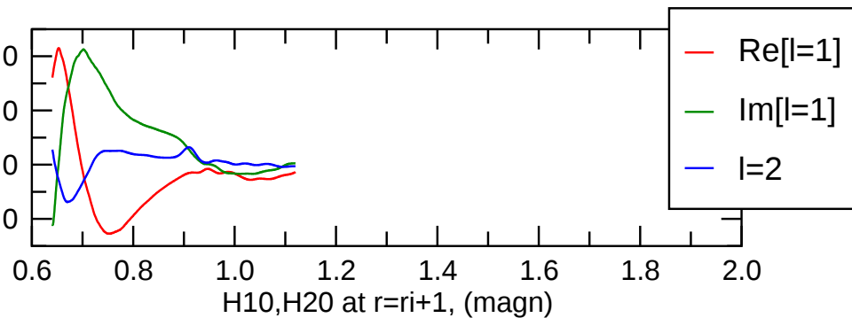
pol(m=1) magn.
