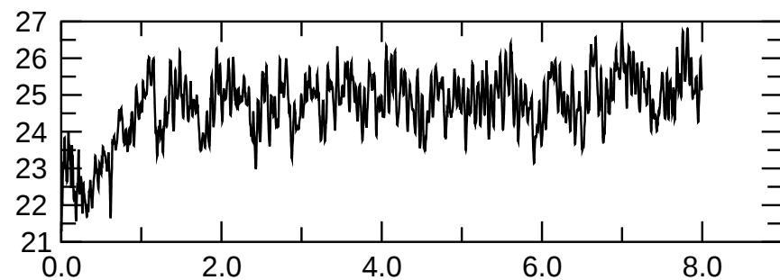
m=2 kin.
