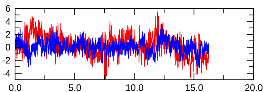
pol(m=0) magn.
