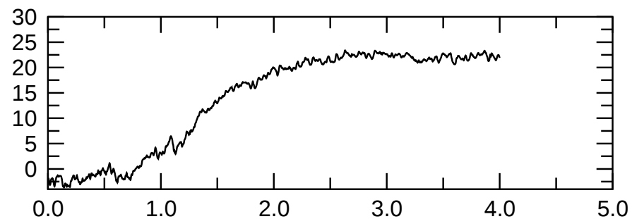
m=2 kin.
