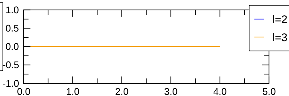
pol(m=0) magn.
