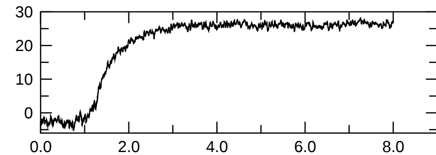
m=2 kin.
