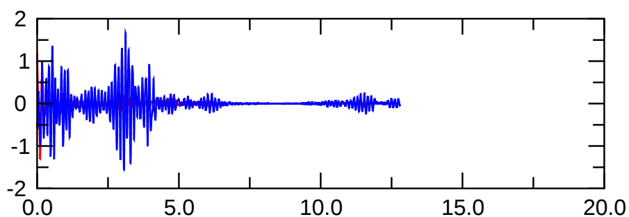
pol(m=0) magn.
