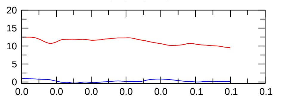
pol(m=0) magn.
