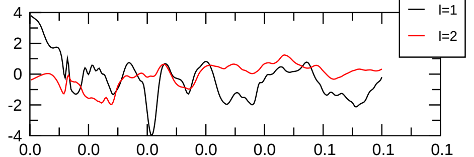
pol(m=2) magn.
