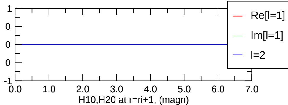
pol(m=1) magn.
