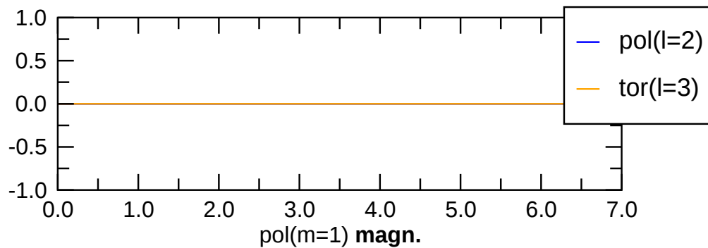
m=2 kin.
