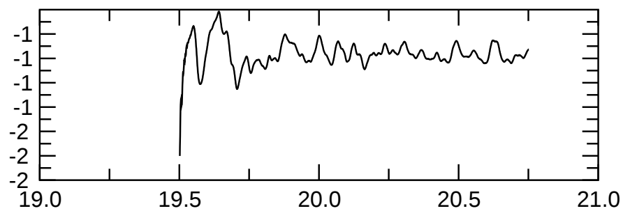
m=2 kin.
