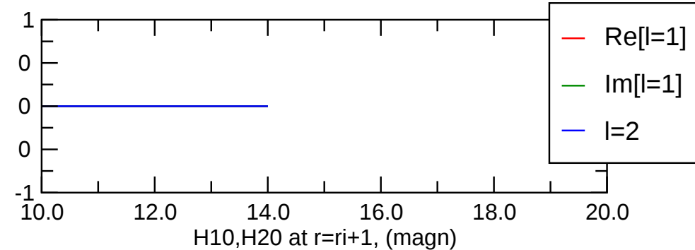
pol(m=1) magn.
