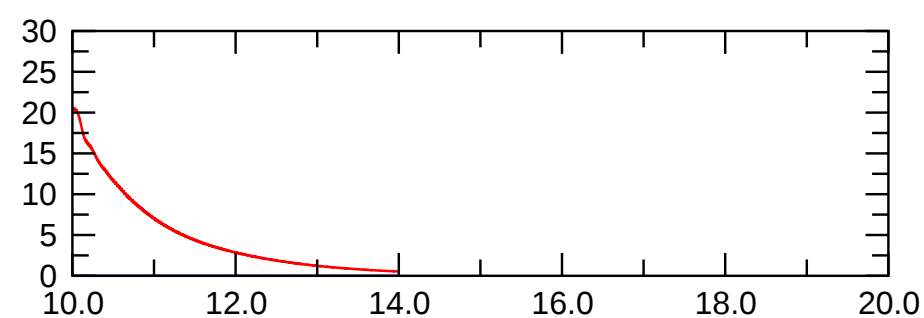
pol(m=0) magn.
