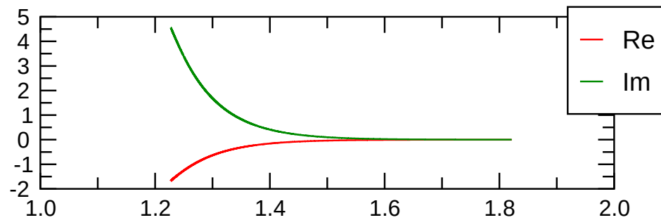
pol( l=1, m=1 ) kin.
