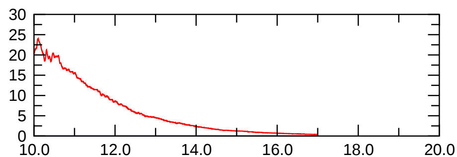
pol(m=0) magn.
