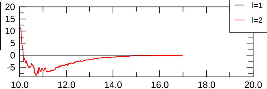
pol(m=2) magn.
