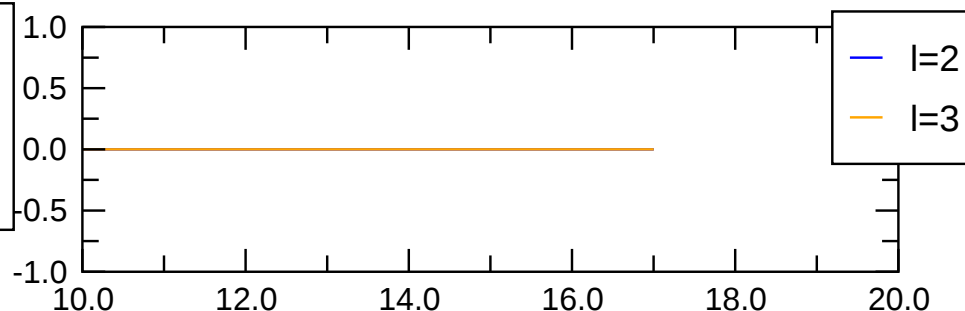
pol(m=0) magn.
