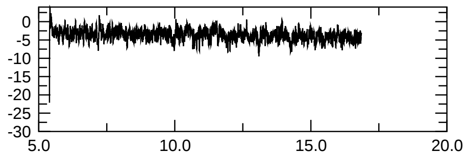
m=2 kin.
