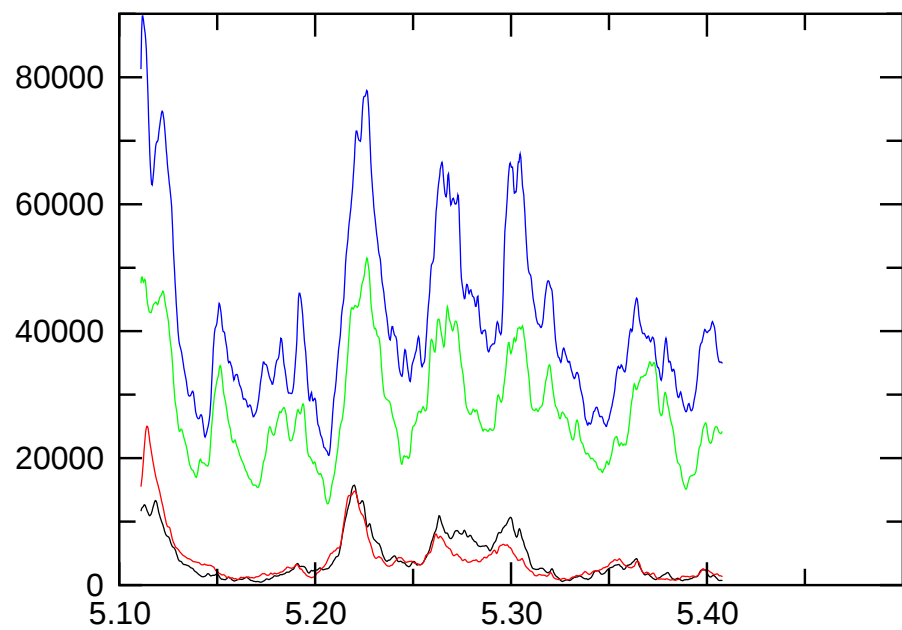
E_{\text{magn,quadr.}}
