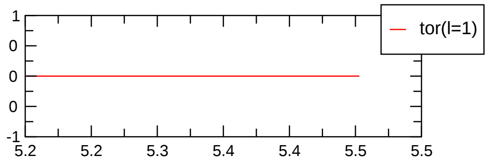
tor(l=1,m=1) kin.
