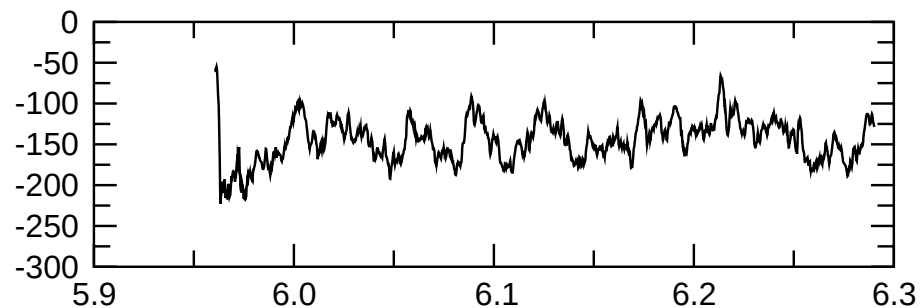
m=2 kin.
