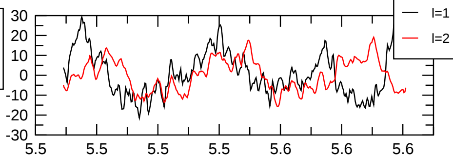
pol(m=2) magn.
