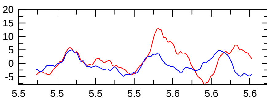
pol(m=0) magn.
