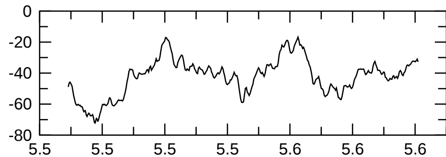
m=2 kin.
