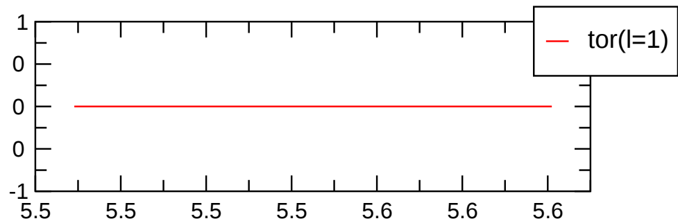
tor(l=1,m=1) kin.
