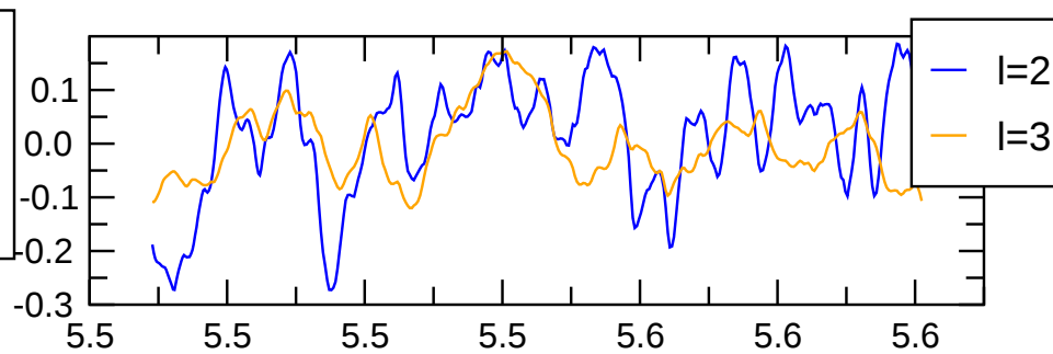
pol(m=0) magn.
