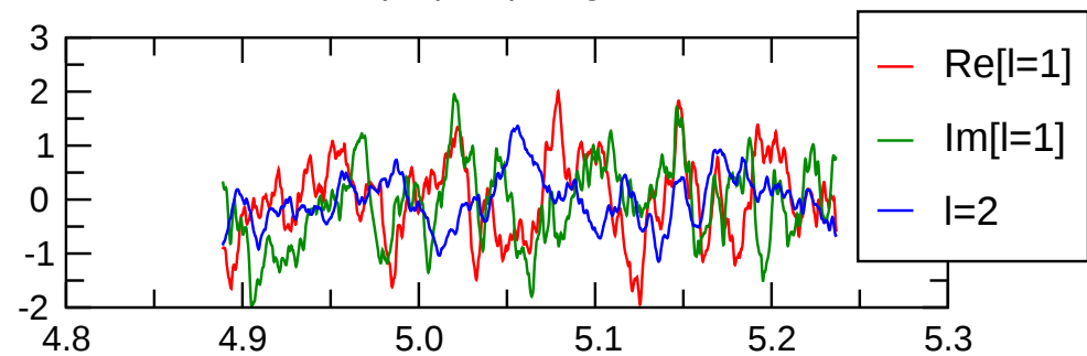
tor(l=1,m=1) kin.
