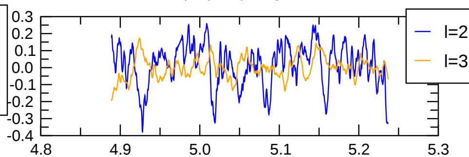
pol(m=0) magn.
