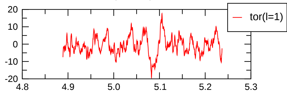
tor(l=1,m=1) kin.
