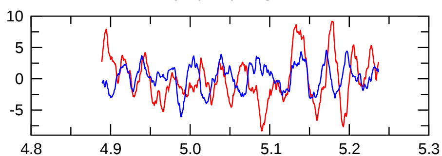
pol(m=0) magn.
