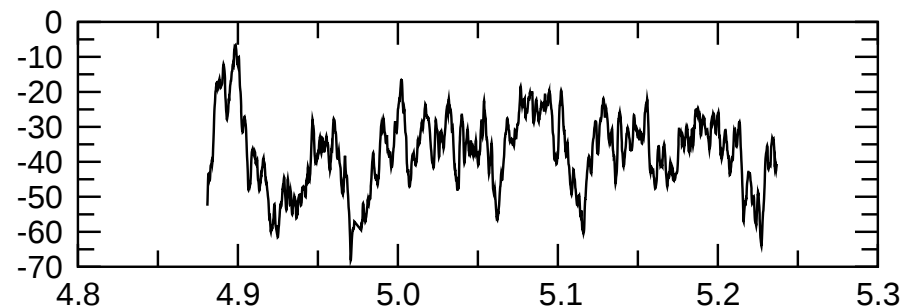
m=2 kin.
