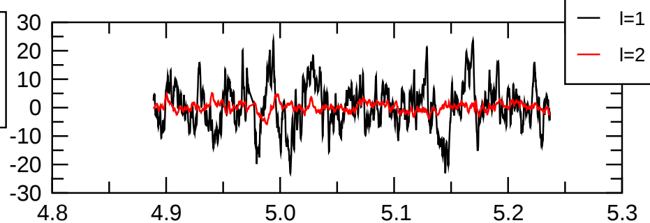
pol(m=2) magn.
