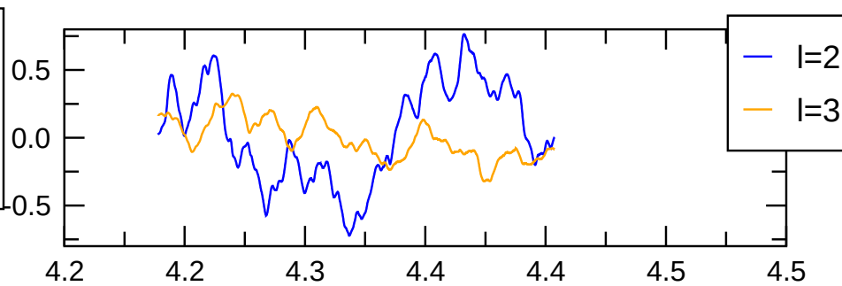
pol(m=0) magn.
