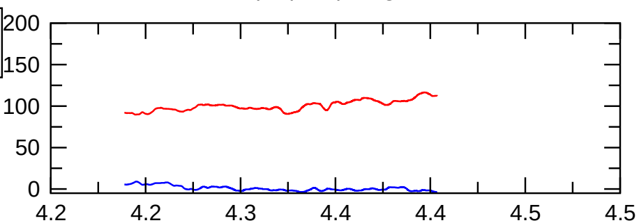
pol(m=0) magn.
