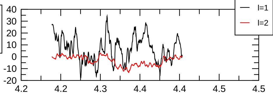
pol(m=2) magn.
