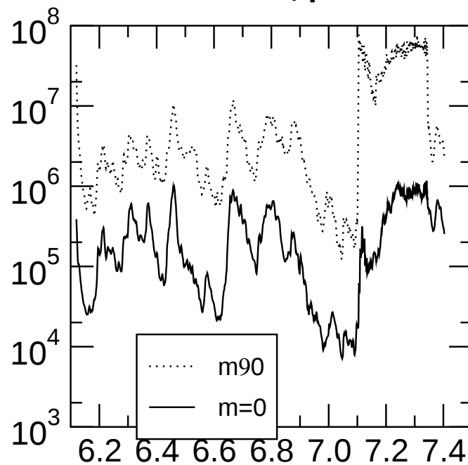
ohmic diss., poloidal
