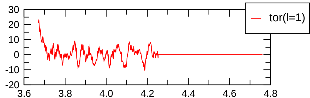
tor(l=1,m=1) kin.
