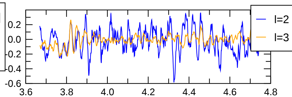
pol(m=0) magn.
