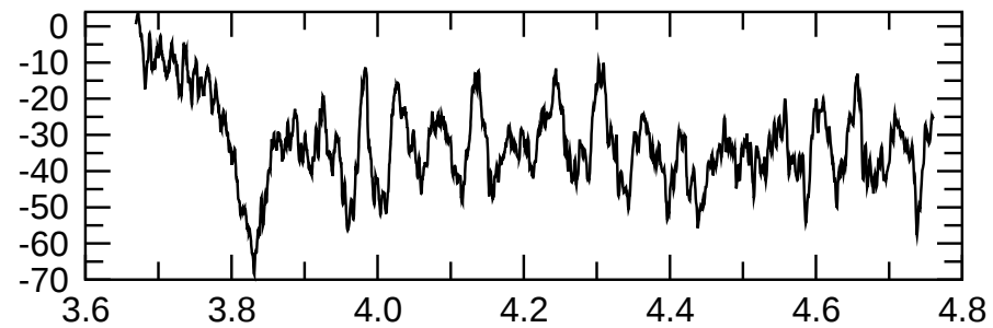
m=2 kin.
