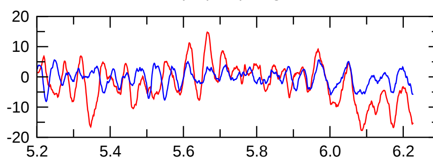
pol(m=0) magn.
