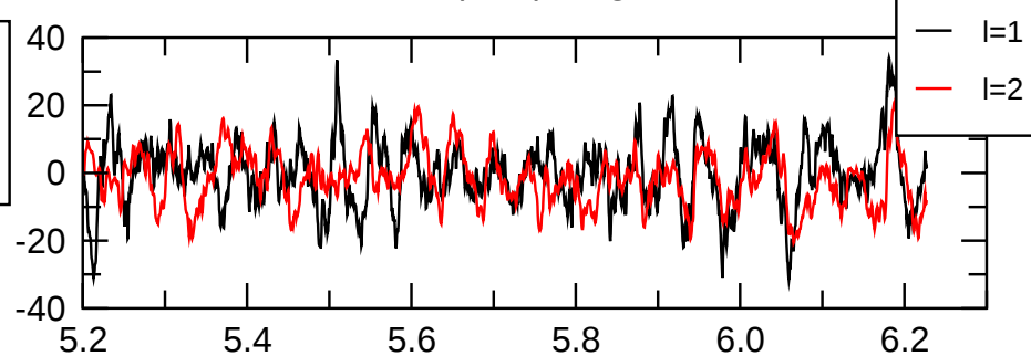
pol(m=2) magn.
