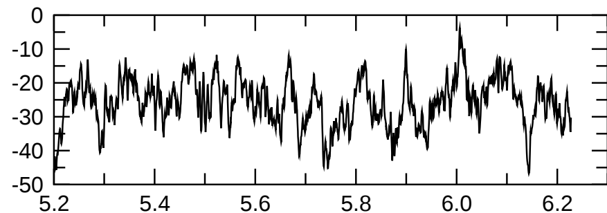
m=2 kin.
