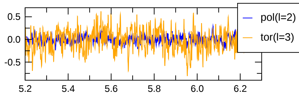
pol(m=1) magn.
