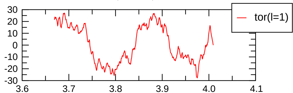
tor( l=1, m=1 ) kin.
