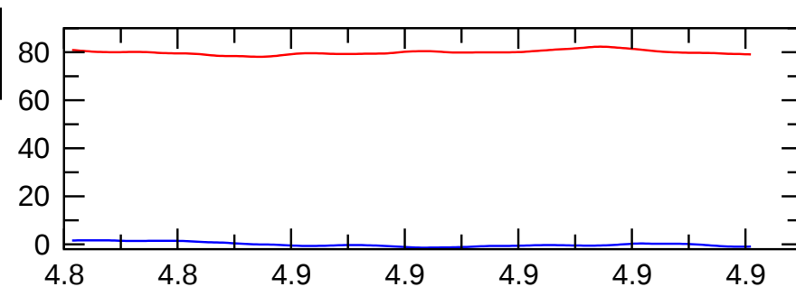
pol(m=0) magn.
