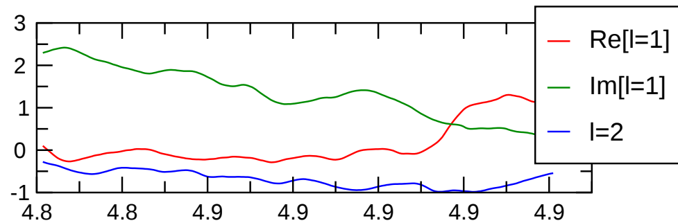
tor(l=1,m=1) kin.
