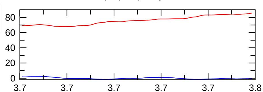
pol( m=0 ) magn.
