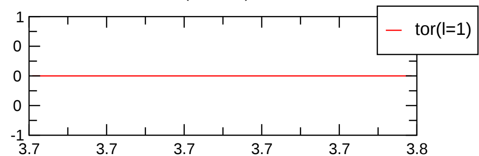
tor( l=1, m=1 ) kin.
