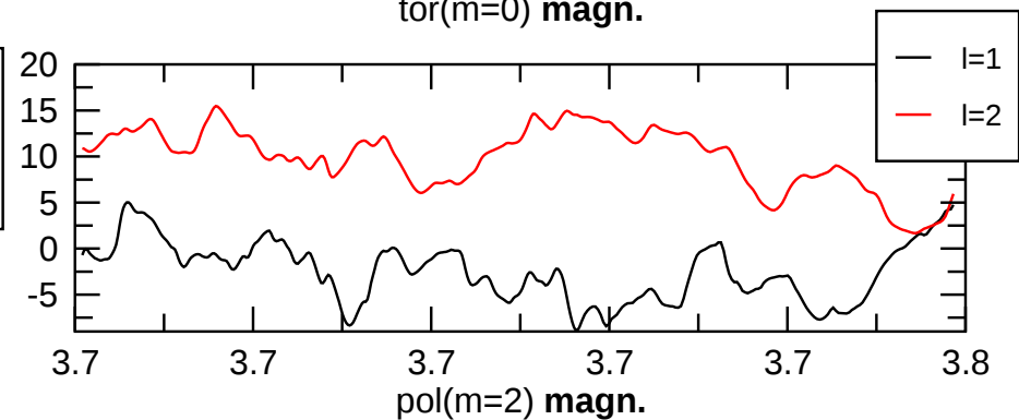
tor( m=0 ) magn.
