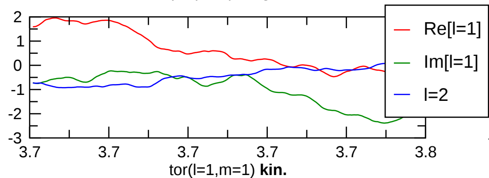
pol( m=1 ) magn.
