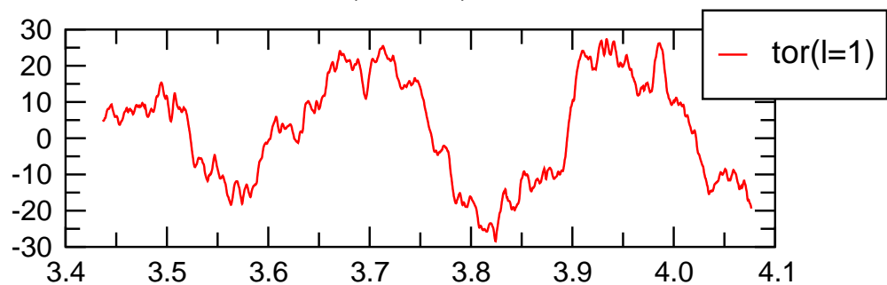
tor(l=1,m=1) kin.
