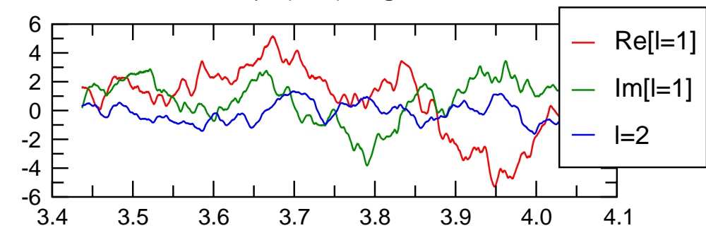
tor(l=1,m=1) kin.
