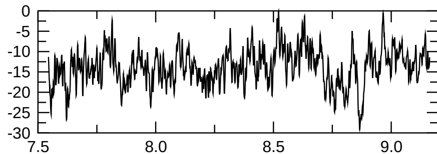
m=2 kin.
