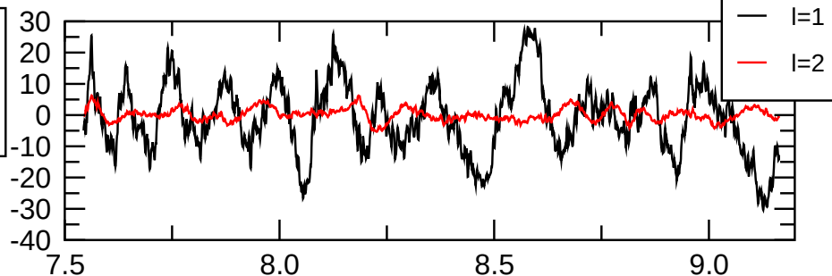
pol(m=2) magn.
