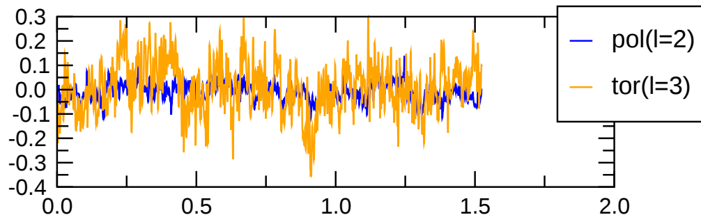
pol( m=1 ) magn.
