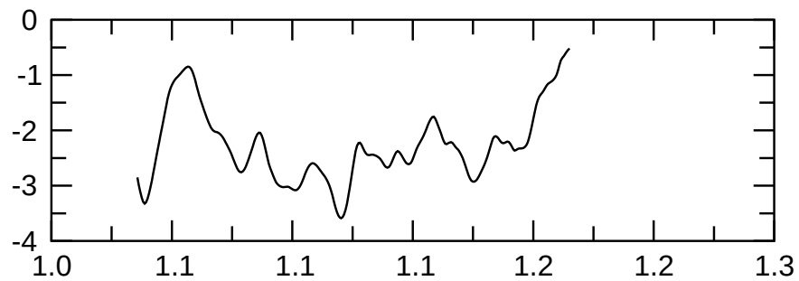
m=2 kin.
