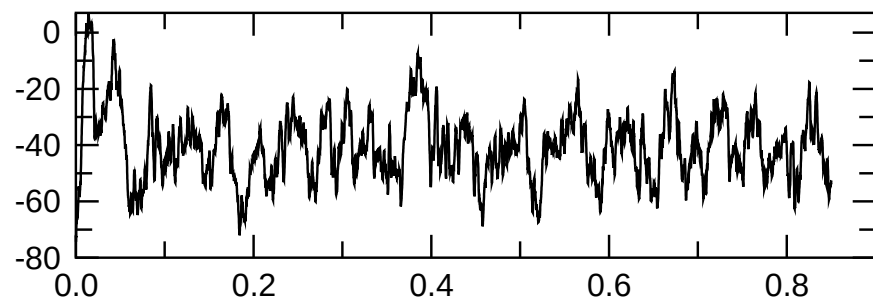
m=2 kin.
