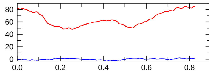
pol(m=0) magn.
