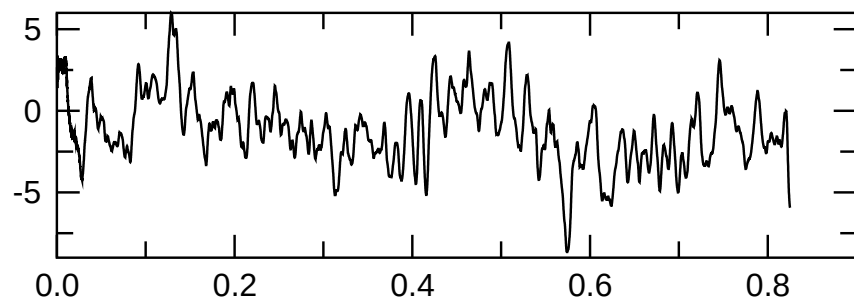
m=2 kin.
