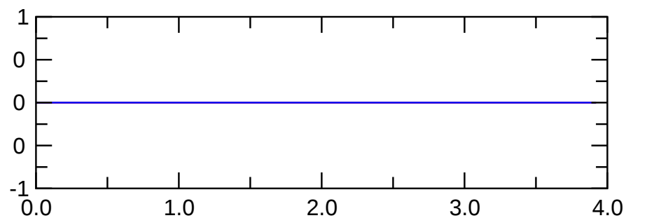
pol(m=0) magn.
